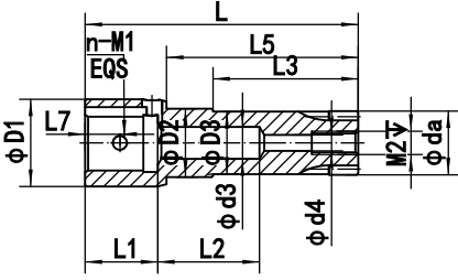
B型特制输入齿轮轴
